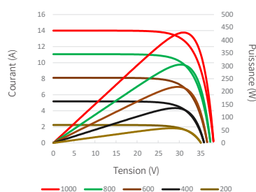
Courbes courant-tension et puissance-tension (430W)
